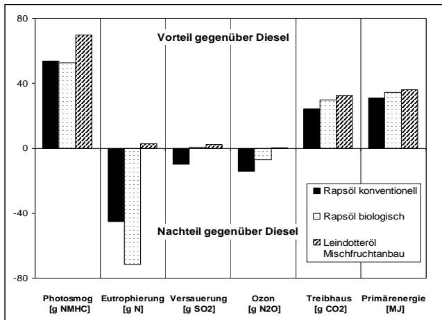
Abb. 1: Ökologischer Vergleich von Dieseldieselkraftstoff mit dezentral hergestellten, kaltgepressten Pflanzenölen (nach: SERGIS-CHRISTIAN & BROWERS 2005).
