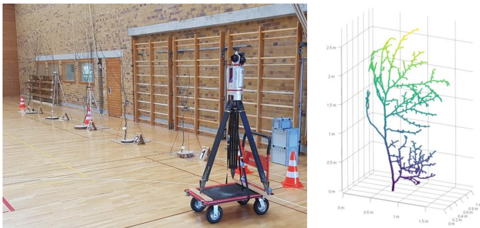
Abb. 16: Auf Rollwagen montierter terrestrische Laserscanner mit Versuchsbäumen im Hintergrund (links) daneben ein QSM eines gescannten Astes (rechts).
