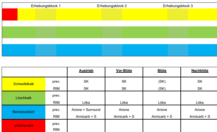
Abb. 2: Anordnung der Verfahren und der Erhebungsblöcke (schraffiert, oben) und Einsatzstrategie für die Biofungizide gegen Birnenschorf im Versuch 2017 (unten)
