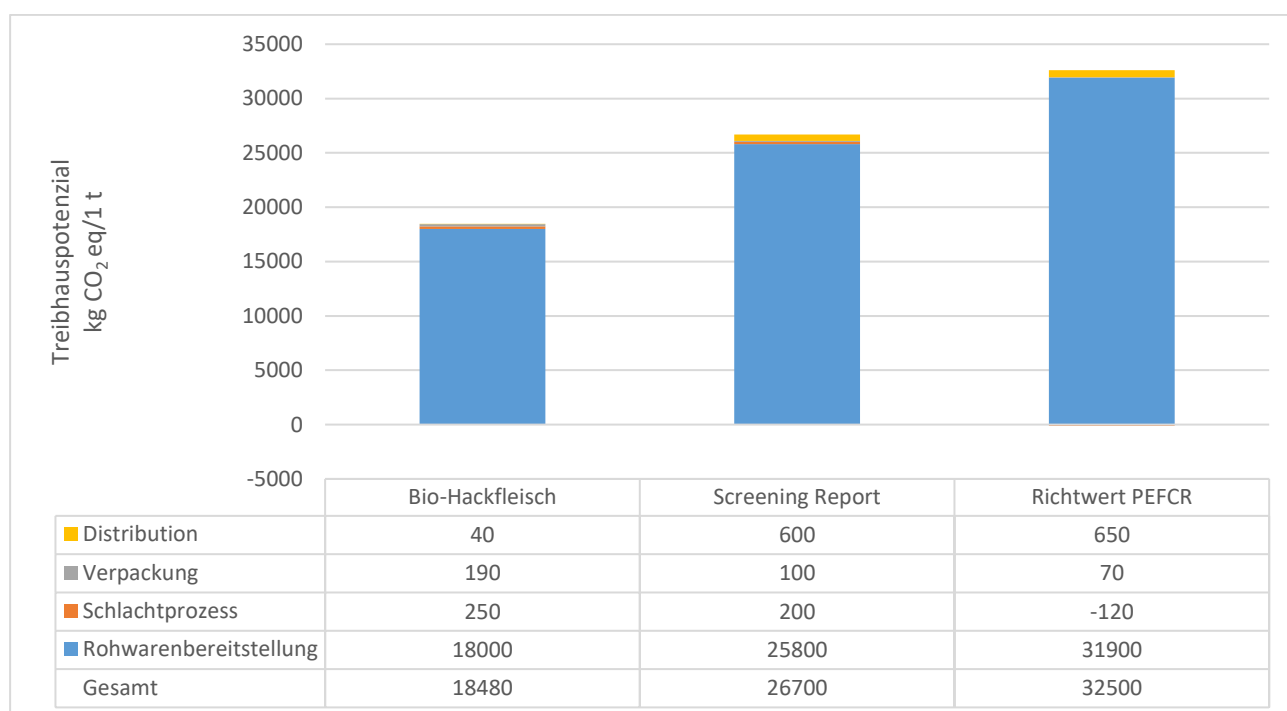
Abbildung 12: Vergleich Treibhauspotenzial des Bio-Hackfleischs mit dem Richtwert der PEFCR und dem Screening Report pro 1 t Fleisch
