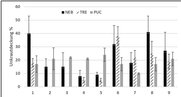
Abbildung 1: Unkrautdeckungsgrad (%) in Neu-Eichenberg (NEB), Trenthorst (TRE) und Puch (PUC) bei Reihenschluss des Maises der Varianten mit 75 cm Reihenabstand, Jahr 2020. 1= Kontrolle, 2= EK WE/Tri+DS, 3=EK Wi/Ro+DS; 4=EK WE/Tri+BB, 5=EK Wi/Ro+BB; 6=WE gewalzt, 7=WE/Tri gewalzt, 8= Wi gewalzt, 9= Wi/Ro gewalzt. Varianten 1-5 mit mechanischer Unkrautregulierung.
