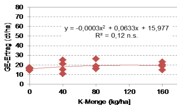
Abbildung 92: GE-Ertrag der Ackerbohnen im Jahr 2002 in Abhängigkeit von der K-Steigerung
