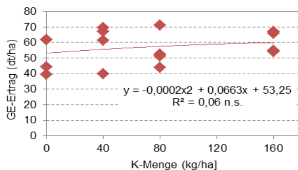
Abbildung 102: GE-Ertrag des Winterweizens im Jahr 2007 in Abhängigkeit von der K-Steigerung
