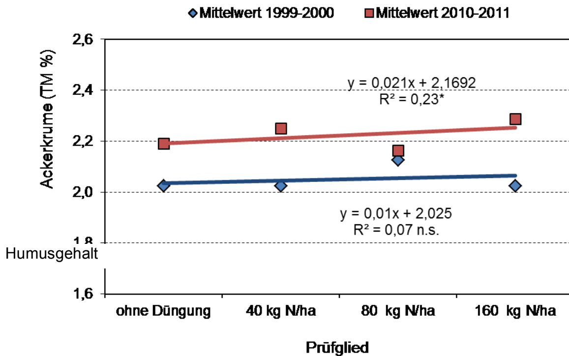
Abbildung 42: Humus-Gehalte in den jeweiligen Düngungsstufen zu Beginn und zum Ende der Versuchsreihe
