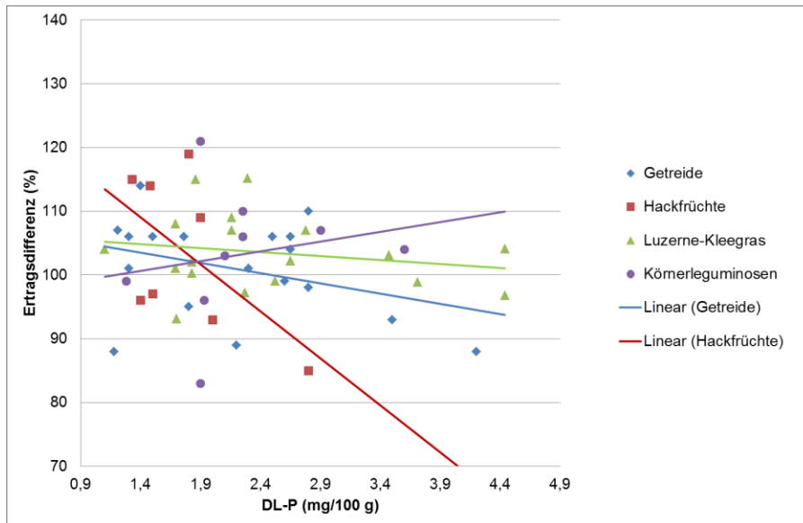
Abbildung 129: Durchschnittliche Ertragswirkung einzelner Fruchtartengruppen durch zusätzliche mineralische P-Düngung (ohne Düngung = 100 %) in Abhängigkeit von den DL-P-Bodengehalten ermittelt durch einfache Regressionsanalysen
