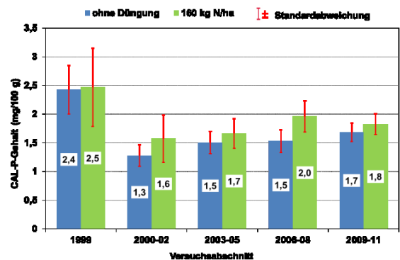
Abbildung 35: Einfluss der organischen Düngung auf die CAL-P-Gehalte des Bodens in den verschiedenen Versuchsabschnitten
