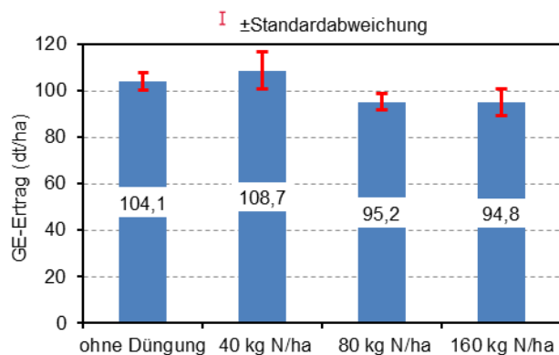
Abbildung 26: Mittlerer GE-Ertrag des Luzerne-Klee-grases in 2011 nach organischer Düngung
