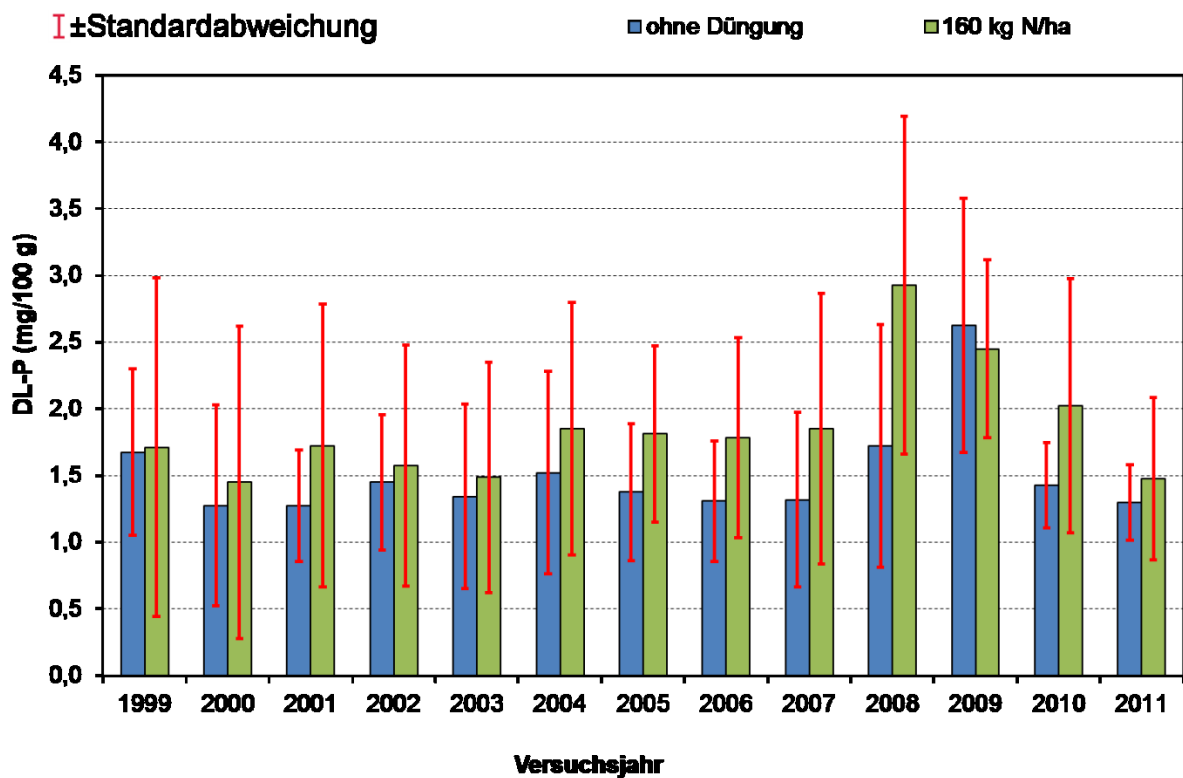
Abbildung 33: Ergebnisse der jährlichen Bodenuntersuchung (inklusive Standardabweichung der Mittelwerte) auf die DL-P-Gehalte in den Varianten ohne Düngung und mit 160 kg N/ha als organische Dünger
