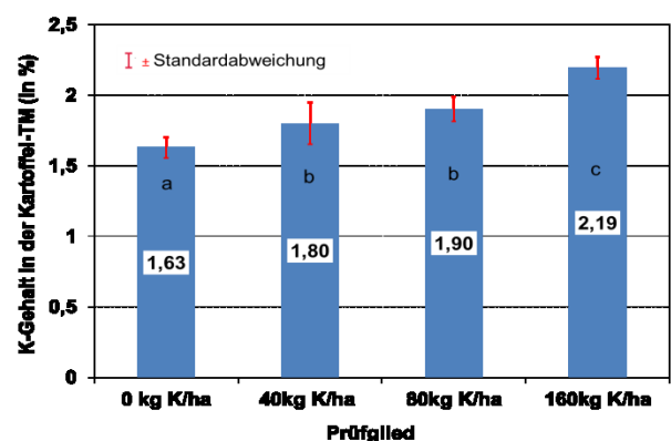
Abbildung 114: K-Gehalte in der TM der Kartoffeln in der K-Steigerungsreihe des Jahres 2001
