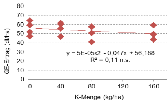
Abbildung 106: GE-Ertrag der Wintergerste in 2009 in Abhängigkeit von der K-Steigerung
