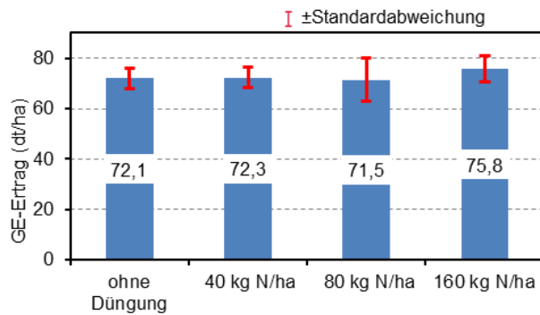
Abbildung 14: Mittlerer GE-Ertrag des Luzerne-Klee grasses in 2005 nach organischer Düngung
