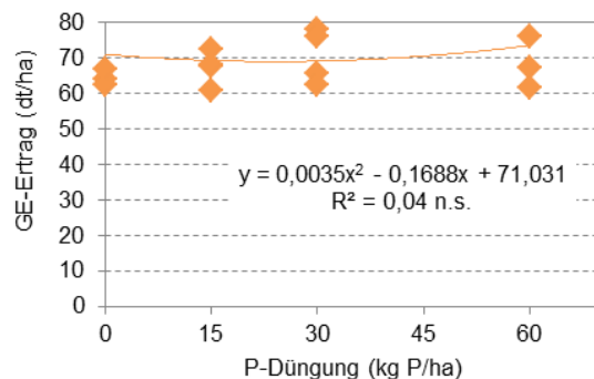
Abbildung 58: GE-Ertrag des Luzerne-Klee-grases in 2004 in Abhängigkeit von der P-Steigerung
