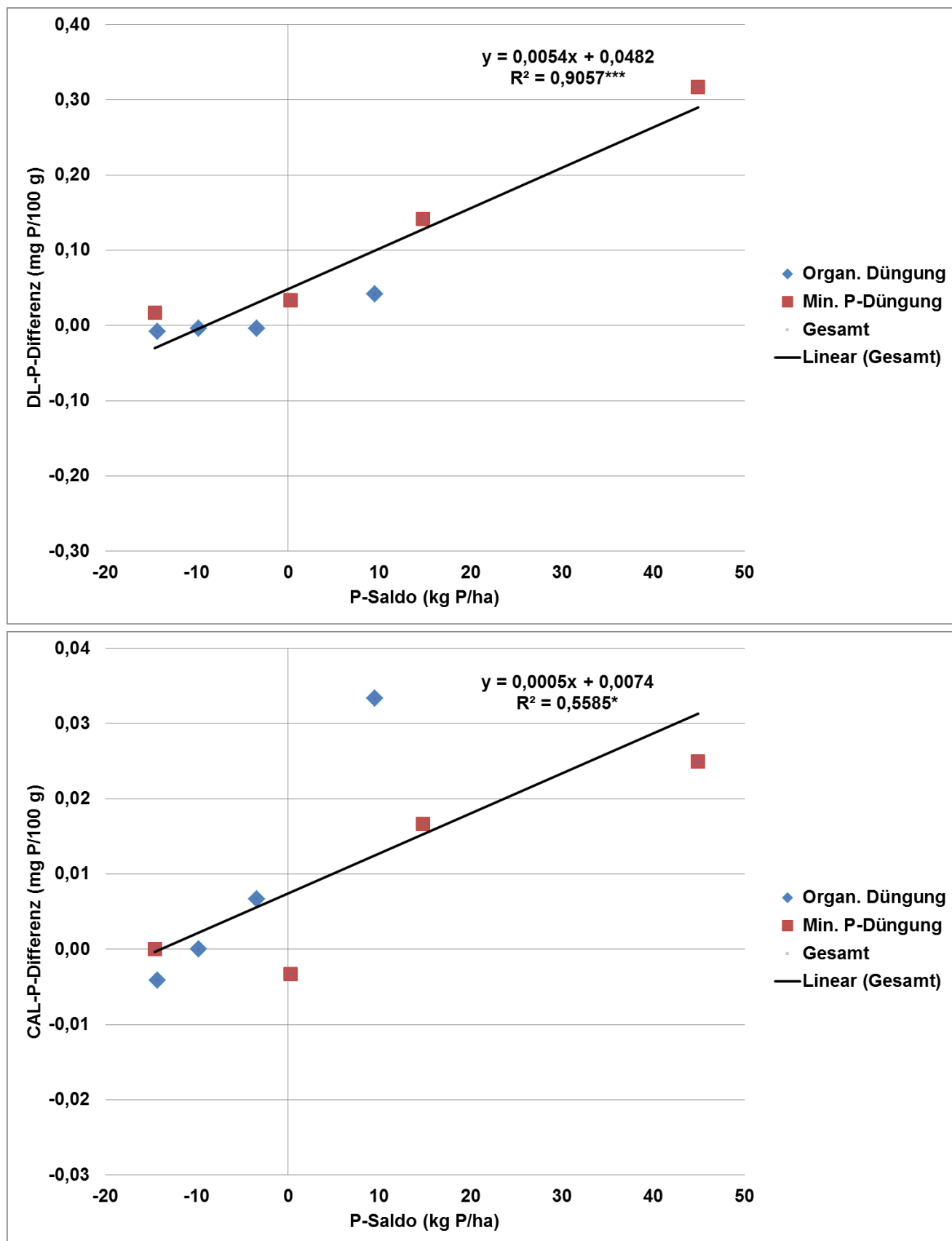
Abbildung 125: Einfluss der P-Schlagsalden auf die jährliche Veränderung der DL- und CAL-löslichen P-Gehalte des Bodens in Folge steigender organischer und mineralischer P-Düngung
