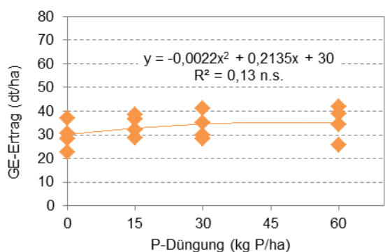
Abbildung 52: GE-Ertrag der Kartoffeln des Jahres 2001 in Abhängigkeit von der P-Steigerung
