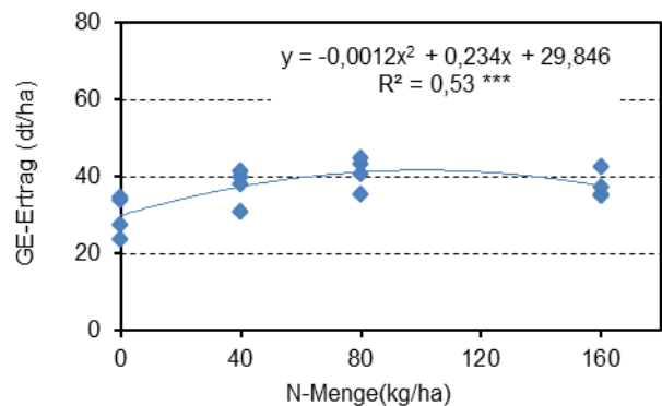
Abbildung 7: GE-Ertrag der Kartoffeln im Jahr 2001 in Abhängigkeit vom N-Einsatz aus organischer Düngung
