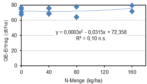
Abbildung 15: GE-Ertrag des Luzerne-Klee grasses im Jahr 2005 in Abhängigkeit vom N-Einsatz aus organischer Düngung
