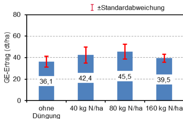
Abbildung 10: Mittlerer GE-Ertrag der Wintergerste nach organischer Düngung im Jahr 2003
