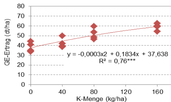
Abbildung 100: GE-Ertrag der Kartoffeln im Jahr 2006 in Abhängigkeit von der K-Steigerung
