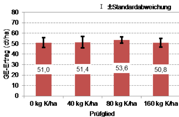
Abbildung 87: Mittlerer GE-Ertrag des Winterweizens im Jahr 2000 in der K-Steigerungsreihe
