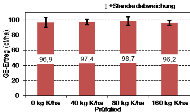
Abbildung 109: Mittlerer GE-Ertrag an Luzerne-Klee-gras im Jahr 2011 in der K-Steigerungsreihe
