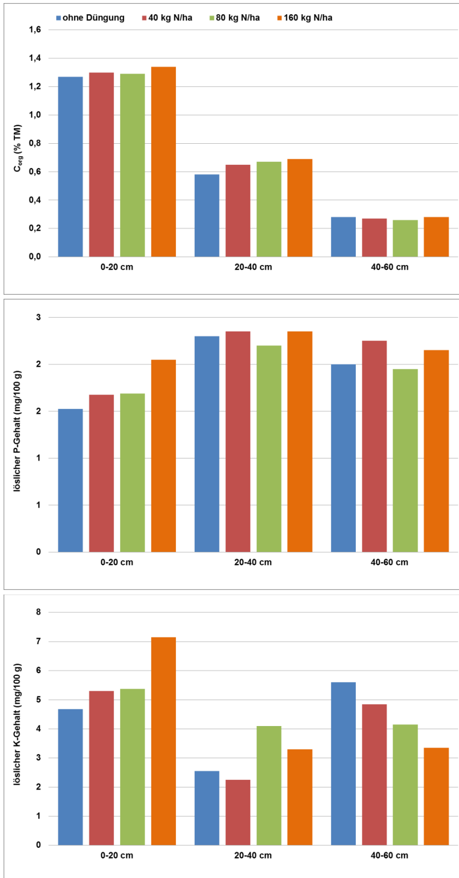
Abbildung 48: Einfluss der organischen Düngung auf die C_{org} -Gehalte (oben) sowie die löslichen P-Gehalte (Mitte) und K-Gehalte (unten) in der Ackerkrume und im Untergrund bis 60 cm Bodentiefe im Jahr 2011
