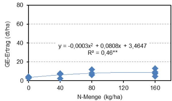
Abbildung 21: GE-Ertrag der Ackerbohnen in 2008 in Abhängigkeit vom N-Einsatz aus organischer Düngung
