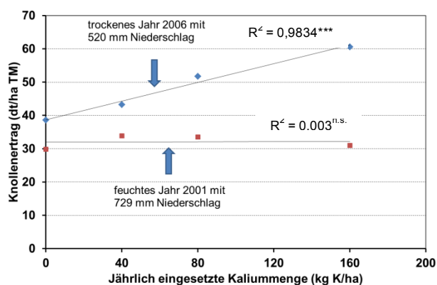
Abbildung 113: Wirkung des gesteigerten Kaliumumsatzes auf den Trockenmasseertrag von Kartoffeln in den Jahren 2001 und 2006.
