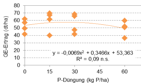
Abbildung 64: GE-Ertrag des Winterweizens im Jahr 2007 in Abhängigkeit von der P-Steigerung
