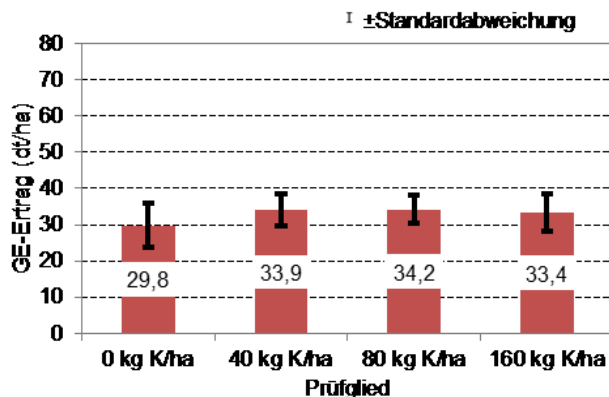
Abbildung 89: Mittlerer GE-Ertrag der Kartoffeln des Jahres 2001 in der K-Steigerungsreihe
