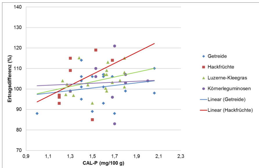
Abbildung 130: Durchschnittliche Ertragswirkung einzelner Fruchtartengruppen durch zusätzliche mineralische P-Düngung (ohne Düngung = 100 %) in Abhängigkeit von den CAL-P-Bodengehalten ermittelt durch einfache Regressionsanalysen
