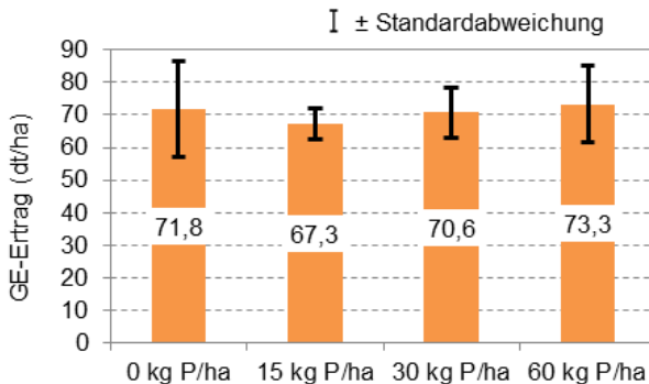
Abbildung 57: Mittlerer GE-Ertrag des Luzerne-Klee-grases im Jahr 2004
