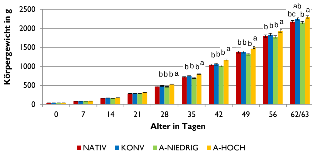
Abbildung 12: Körpergewichtsentwicklung des Fütterungsversuches von Masthühnern mit der Fermentations-Suspension (LS-Means, \pm SE)
