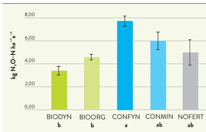
ABB 1: BEWIRTSCHAFTUNG ENTSCHIEDET KLIMARELEVANZ
