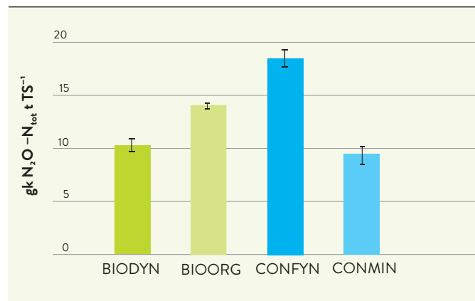
ABB 5: STICKSTOFFEFFIZIENZ DER SYSTEME
