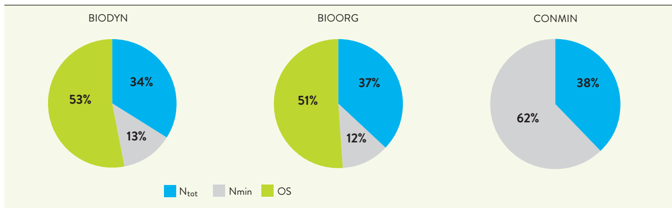
ABB 2: HERKUNFT DES STICKSTOFFS IN DEN VERSCHIEDENEN ANBAUSYSTEMEN
