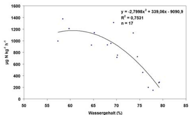
Abbildung 5: Brutto-Nitrifikationsrate im Boden in Abhängigkeit vom Bodenwassergehalt
