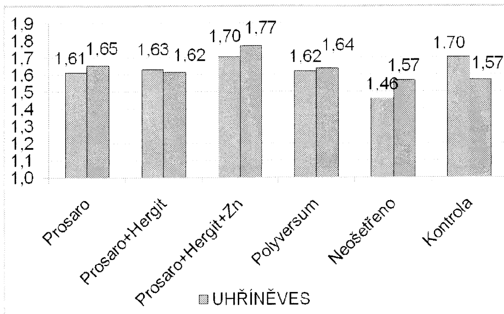
Graf 4: Vliv fungicidního ošetření v butonizaci na výnos máku (t / ha). Uhřetěves, Červený Újezd 2009.
