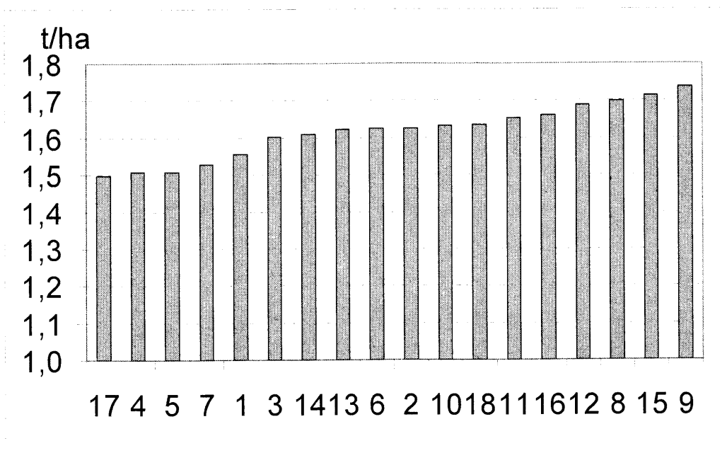
Graf 5: Průměrné výnosy máku (t / ha) u variant pokusu. Uhřetěves, Červený Újezd 2009.
