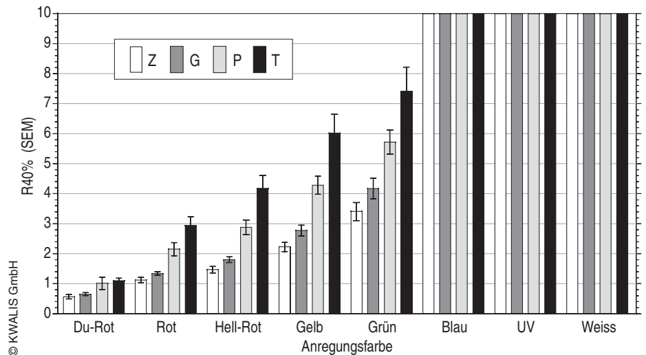
Abb. 3: Das gesamte gemessene Fluoreszenz-Anregungs-Spektrum
