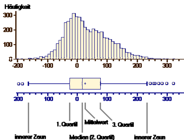
Abbildung 1: Diagrammherleitung Boxplot
