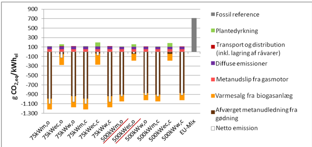
Figur 5.3 Drivhusgasudledning for 12 typer biogasproduktion (biomassegrundlag). Opdelt i bidrag fra forskellige delprocesser og sat i forhold til det elektriske output. Negativ værdi er CO 2 -besparelse og positiv værdi er CO 2 -udledning. Forklaring til det 12 typer: kW angiver størrelsen af anlæggets elektriske produktion (75/500 kW). "m" (manure) står for 90% husdyrgødning og 10% plantebiomasse. "ec" (energy crops) står for 90% plantebiomasse og 10% husdyrgødning. "w" (waste) står for 90% husdyrgødning og 10% husholdningsaffald. "o" (organic) er med økologisk kløvergræs og "c" (conventional) er med konventionel energimajs som plantebiomasse
