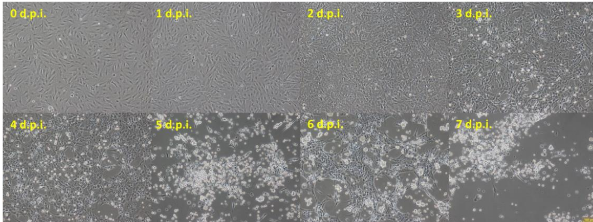
Abbildung 10: Infektionsverlauf des KHV-TP30 in CCB-Zellen
