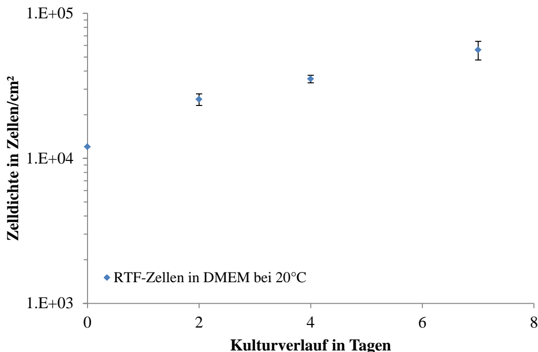
Abbildung 9: Wachstumskurve der RTF-Zellen in DMEM bei 20°C
