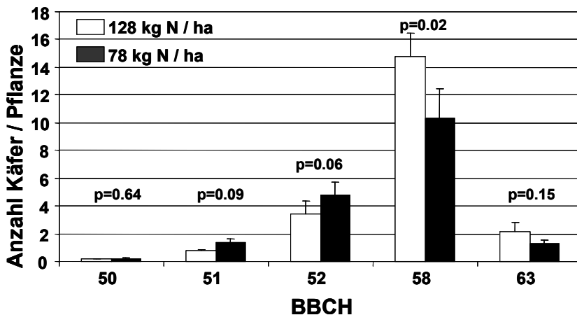
Abbildung 14: Anzahl Rapsglanzkäfer pro Pflanze in den unterschiedlich gedüngten Parzellen in Leibstadt (Statistik two way Anova; BBCH 51: Verfahren F_{1,3}=6.11 , p=0.09 , Block F_{3,3}=1.19 , p=0.44 ; BBCH 5: Verfahren F_{1,3}=7.80 , p=0.06 , Block F_{3,3}=15.78 , p=0.02 ; BBCH 58: Verfahren F_{1,3}=25.52 , p=0.02 , Block F_{3,3}=17.82 , p=0.02 ; BBCH 63: Verfahren F_{1,3}=3.74 , p=0.15 , Block F_{3,3}=3.72 , p=0.15 ).
