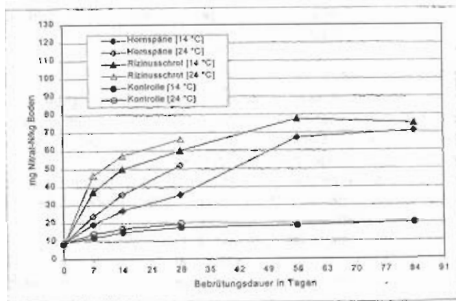
Abb. 1: Nitratansammlung [mg Nitrat-N/kg Boden] durch Umsetzung von Hornspanen und Rizinusschrot im Boden in einem Brutversuch (40 % mWk) bei 14^\circ\text{C} nach 7, 14, 28, 56 und 84 Tagen Bebrütungsdauer und bei 24^\circ\text{C} nach 7, 14 und 28 Tagen Bebrütungsdauer [mWk = maximale Wasserhaltekapazität]
