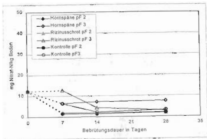
Abb. 2: Nitratansammlung [mg Nitrat-N/kg Boden] durch Umsetzung von Hornspänen und Rizinussschrot im Boden in einem Brutversuch (24 °C) bei Wasserspannungen von pF 2 und pF 3 nach 7, 14 und 28 Tagen Bebrütungsdauer
