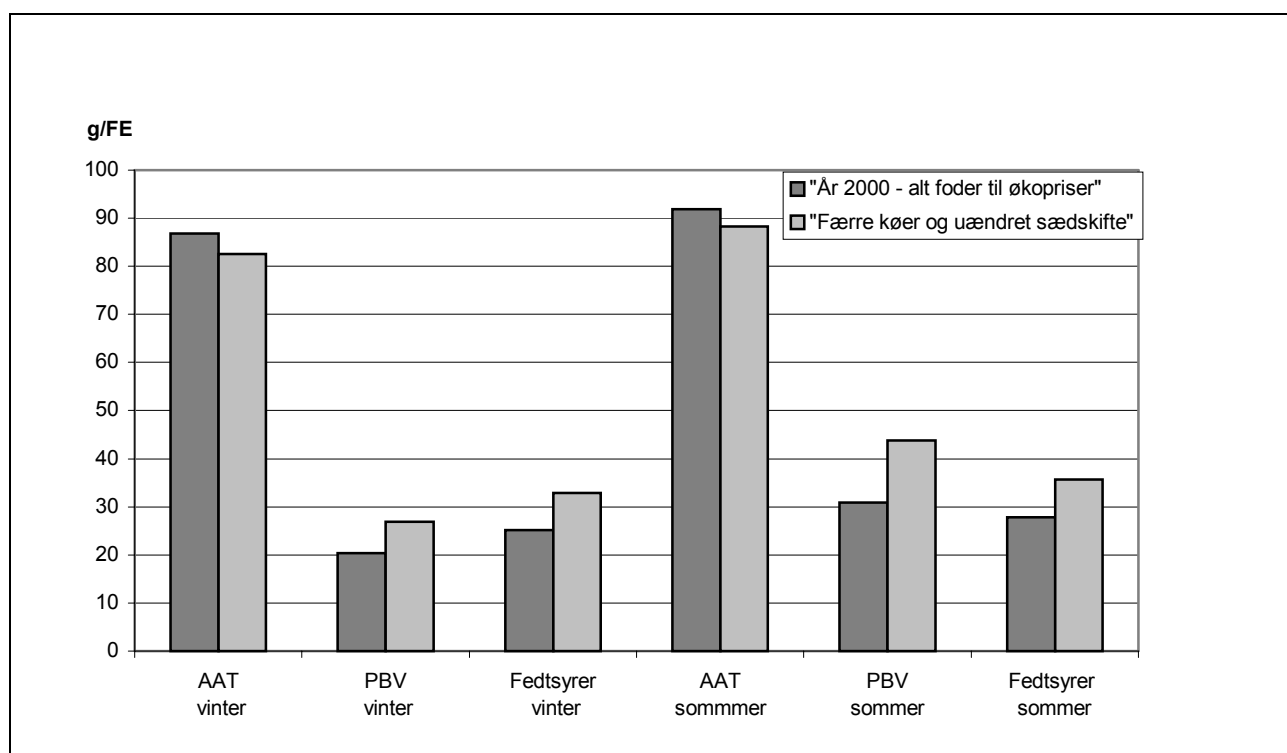
Figur 2 Gennemsnitligt AAT, PVB og fedtsyreindhold i sommer- og vinterfoderrationerne i scenario 1 og 2
