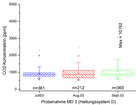
Abbildung 3-189: CO 2 -Konzentration im Haltungssystem D im Mastdurchgang 3
