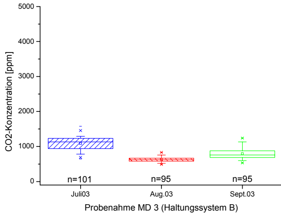
Abbildung 3-169: CO 2 -Konzentration im Haltungssystem B (Abteil 2) im Mastdurchgang 3
