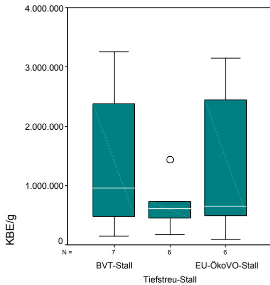
Abbildung 3-53: Stroh, Gesamtschimmelpilze
