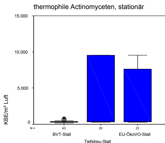
Abbildung 3-4: th.Actinomyceten, stationär
