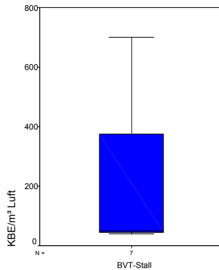
Abbildung 3-66: Flüssigfutter, Coliforme
