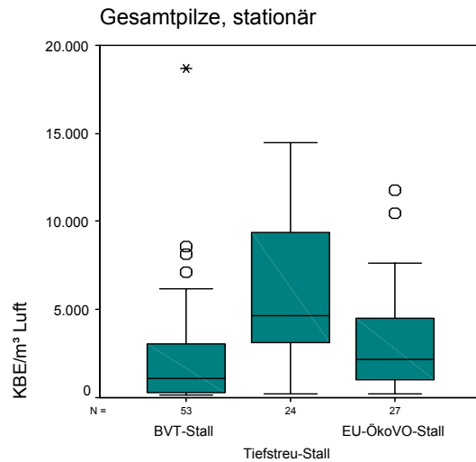
Abbildung 3-2: Gesamtpilze, stationär
