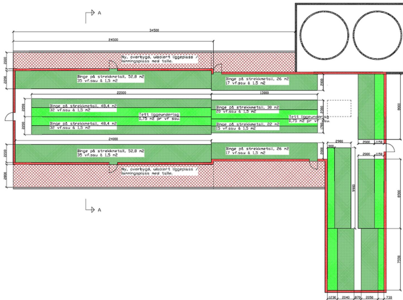
Tegning 1: Plantegning av forslag til løsning, alternativ 2. Tegnet av Knut Hagen ved Norsk Landbruksrådgivning Innlandet.
