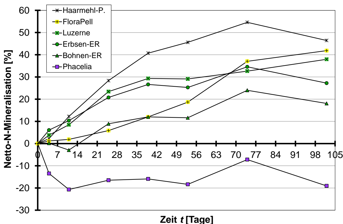
Abb. 2: Verlauf der Netto-N-Mineralisation bei den getesteten Düngern (Mittelwerte über die Wiederholungen)
