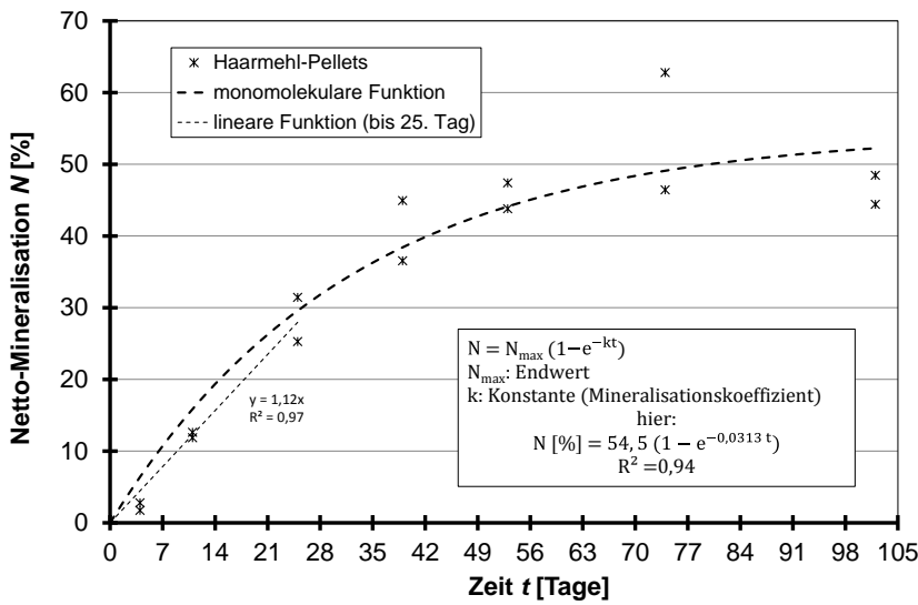
Abb. 3: Verlauf der Netto-N-Mineralisation bei Haarmehl-Pellets
