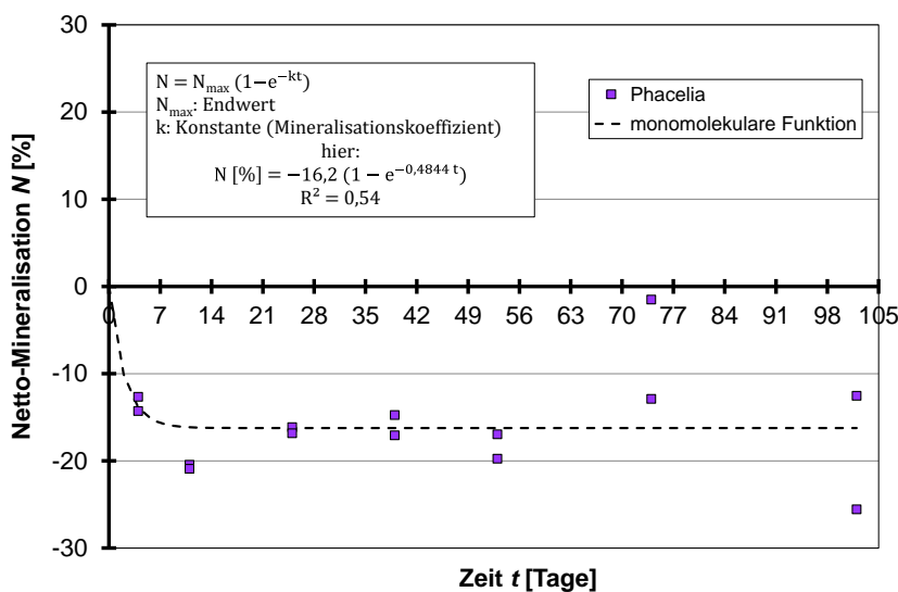
Abb. 8: Verlauf der Netto-N-Mineralisation (hier N-Immobilisation) bei Phacelia
