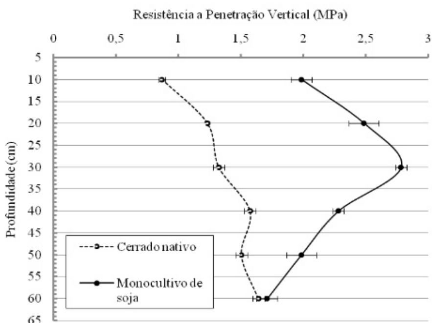
Figura 1. Resistência mecânica do solo à penetração vertical. As barras indicam os valores de erro padrão da média e a sobreposição destas denota a ausência de diferenças entre as médias dos tratamentos, Cáceres-MT, 2009.
